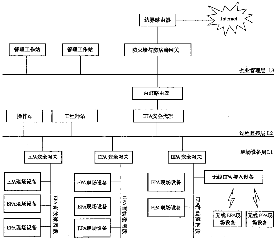
图 1 EPA 网络结构
